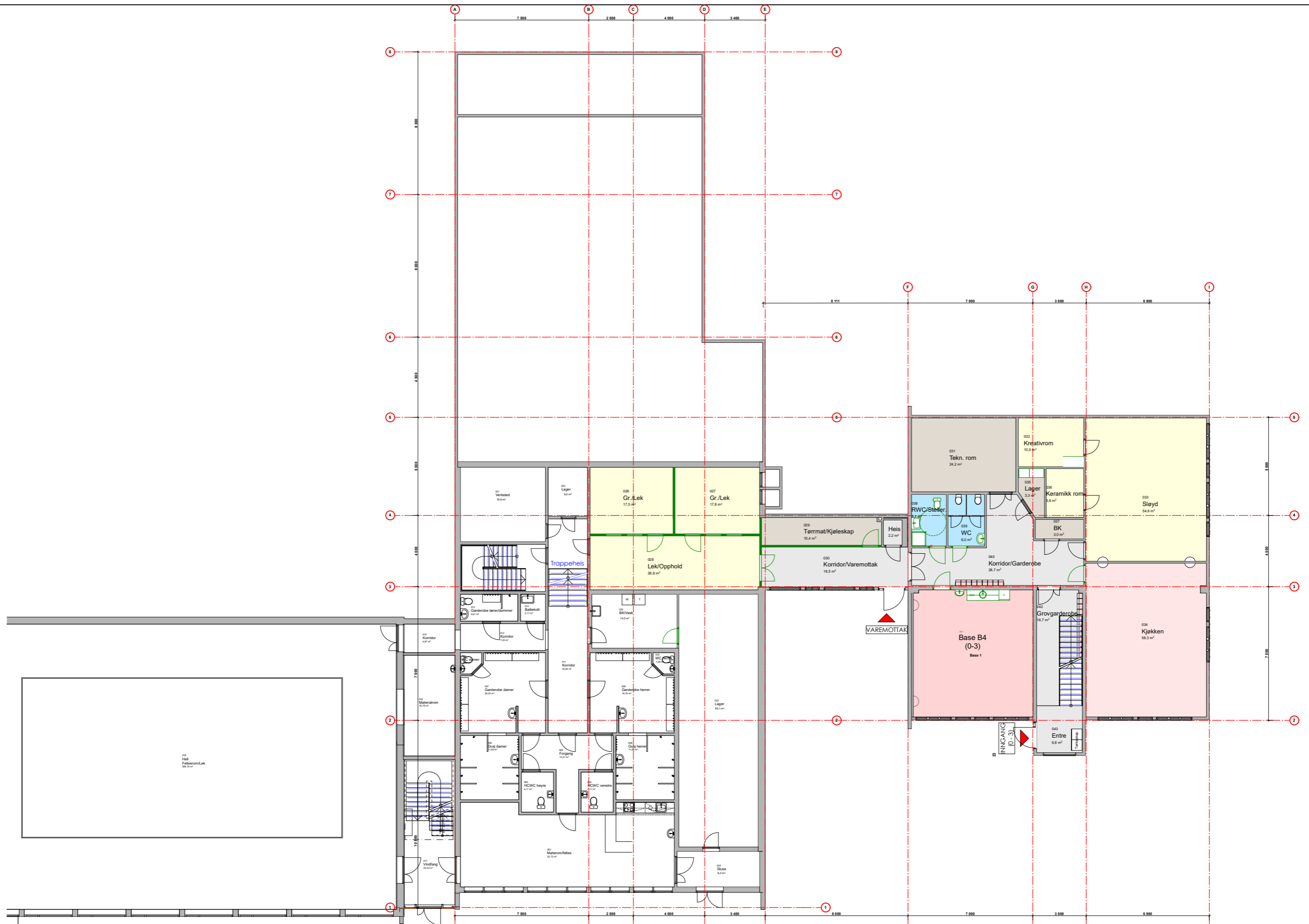
5185672 - Meløy kommune - Ny barnehage Neverdal - Plan U. Etasje - 2018-11-02 - 1:200 -
