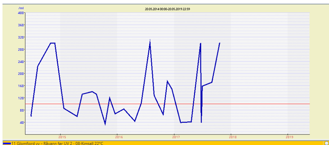
Figur 4-16, viser råvannets innhold av kimfall [CFU/ml]
